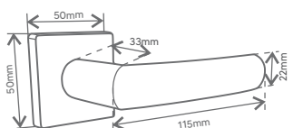
Navis II 09 - Quadrada Grande
