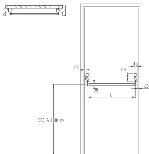
BARRA ANTIPÂNICO PUSH SIMPLES
