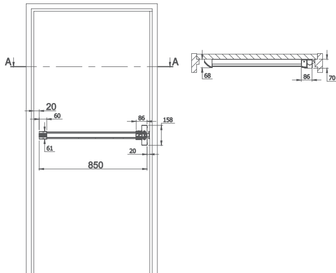
BARRA ANTIPÂNICO TOUCH HORIZONTAL
