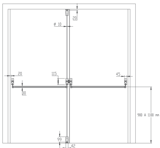
BARRA ANTIPÂNICO PUSH DUPLA
