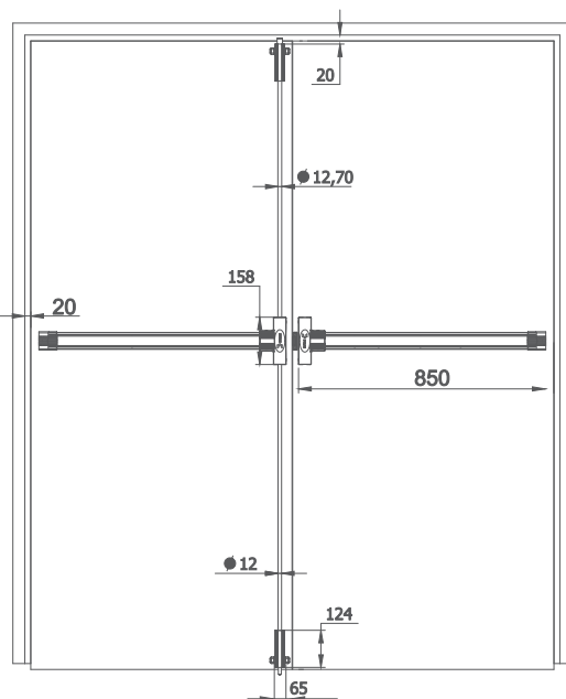
BARRA ANTIPÂNICO TOUCH DUPLA
