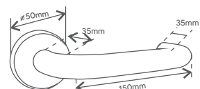
Ceci 01 - Redonda Grande
