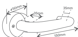
Ceci 10 - Redonda Grande c/ parafuso aparente
