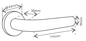
Marine 04 - Redonda pequena
