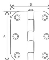
Dobradiça Pino Simples Raio 16 Aço Zincado
