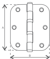
Dobradiça Com Anéis Aço Cromado Raio 16
