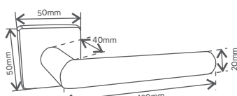
Luck 09 - Quadrada Grande
