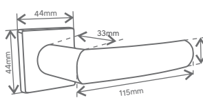
Navis II 07 - Quadrada pequena
