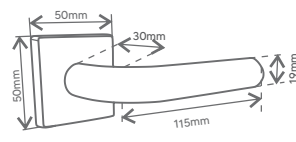
Marine Color 09 - Quadrada Grande
