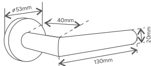
Luck 01 - Redonda Grande
