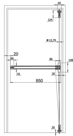
BARRA ANTIPÂNICO TOUCH VERTICAL
