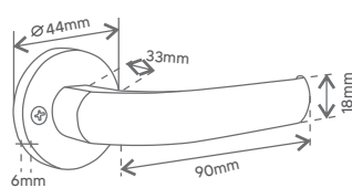
Gol 06 - Redonda Pequena c/ parafuso aparente
