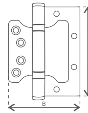
Dobradiça Sobrepor inox Canto Reto
