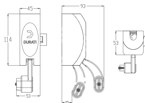
SUPORE P/ BARRA ANTIPÂNICO
