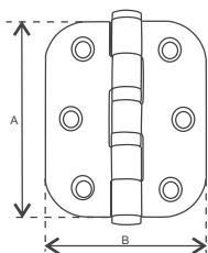
Dobradiça Com Rolamento inox Raio 16
